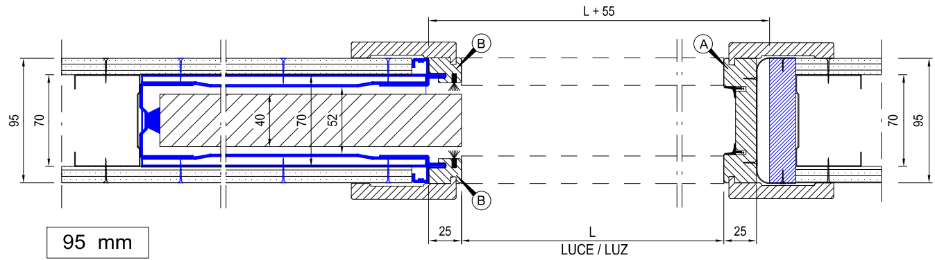
SEZIONE ORIZZONTALE / SECCIÓN HORIZONTAL
