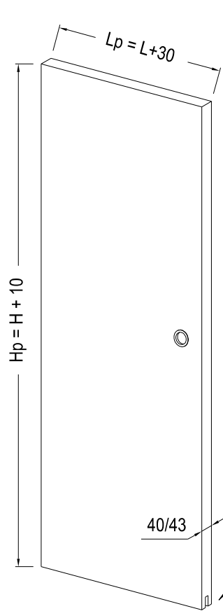
DIMENSIONI PANNELLO - MEDIDAS HOJAS DE PUERTA
