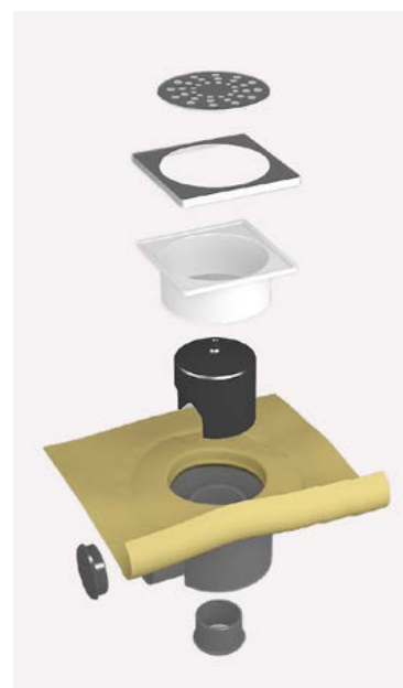
SUMIDERO SIFÓNICO PARA TELA IMPERMEABILIZANTE
