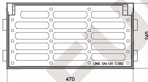
CONJUNTO. VISTA SUPERIOR.
